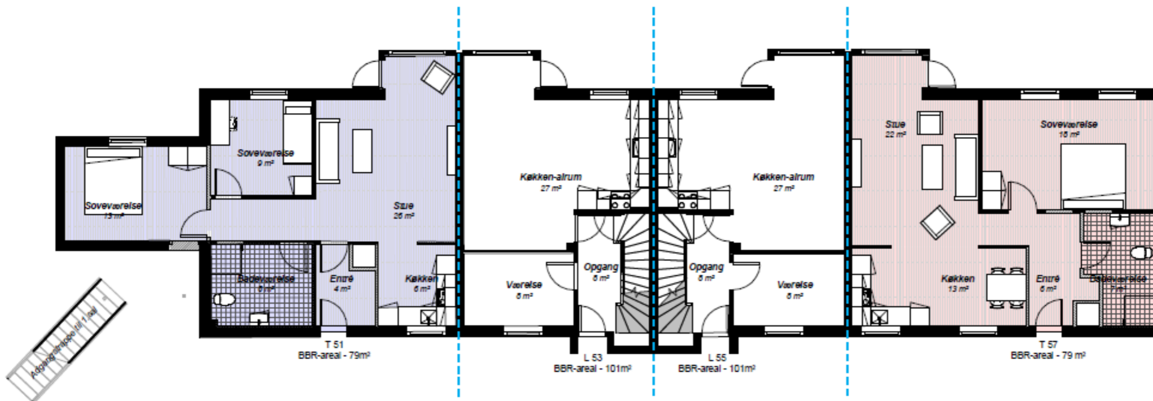
Blok 4 - Stueplan
