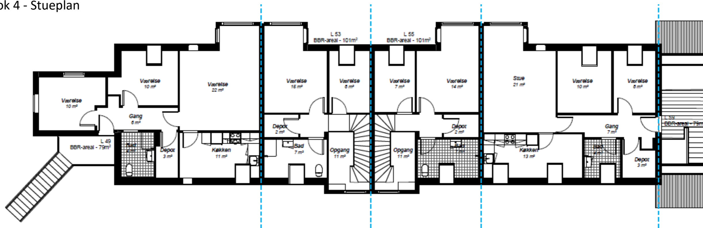
Blok 4- 1. sal
